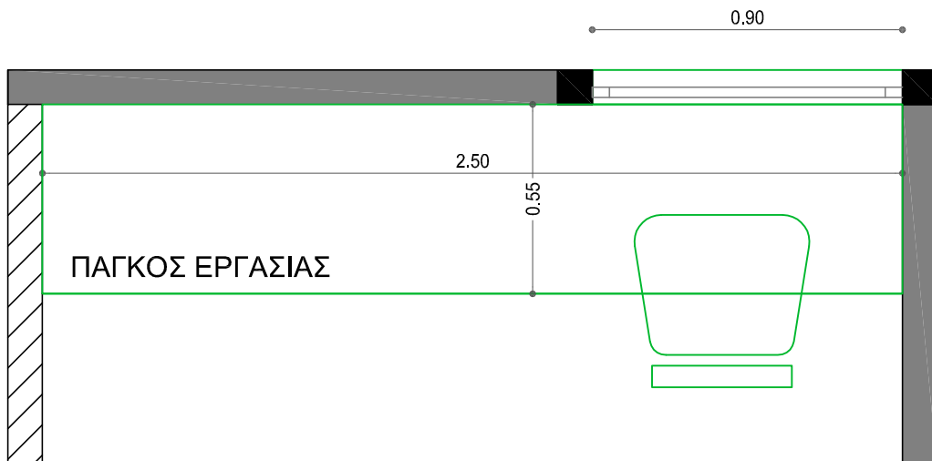
κατοψη - κλ.1/20
