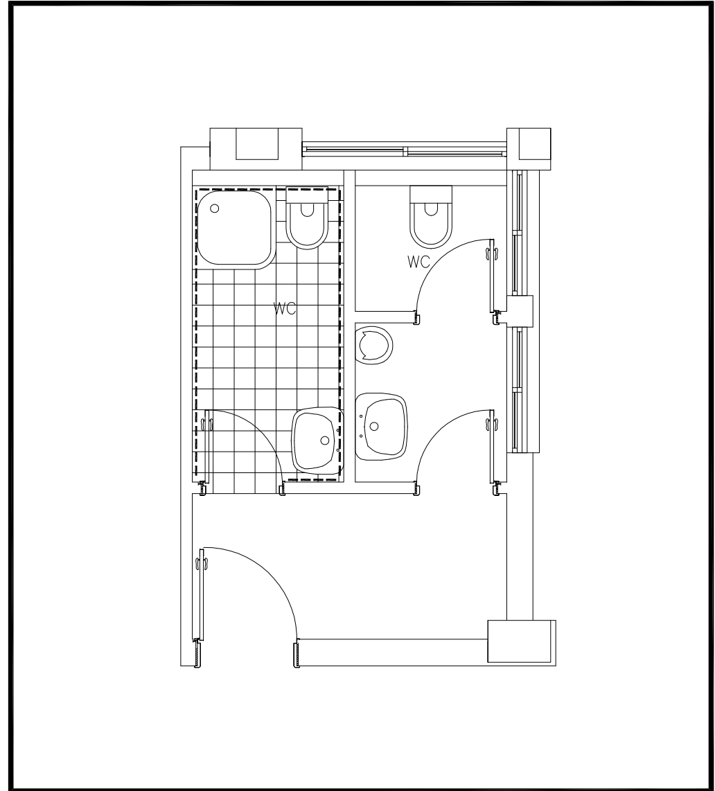
ΠΡΟΤΕΙΝΟΜΕΝΗ ΛΥΣΗ
