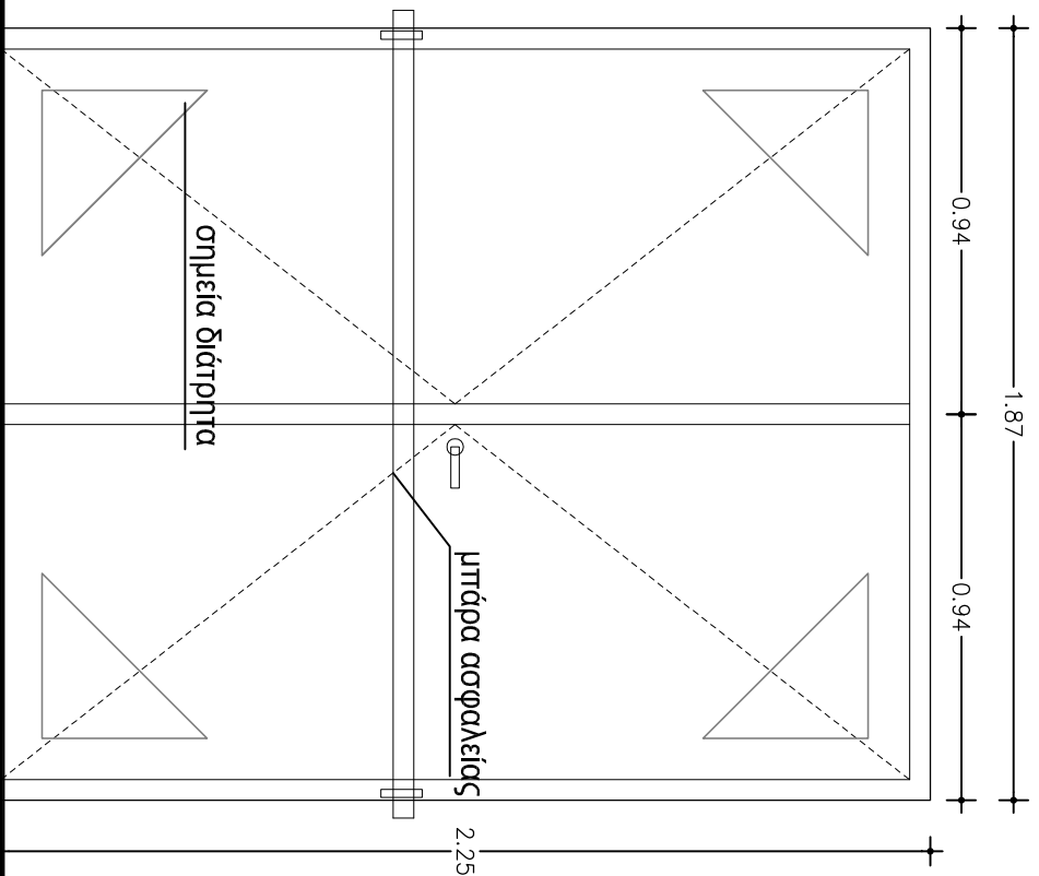
Θ1 : ΔΙΦΩΛΗ ΕΣΩΤΕΡΙΚΗ ΘΥΡΑ
