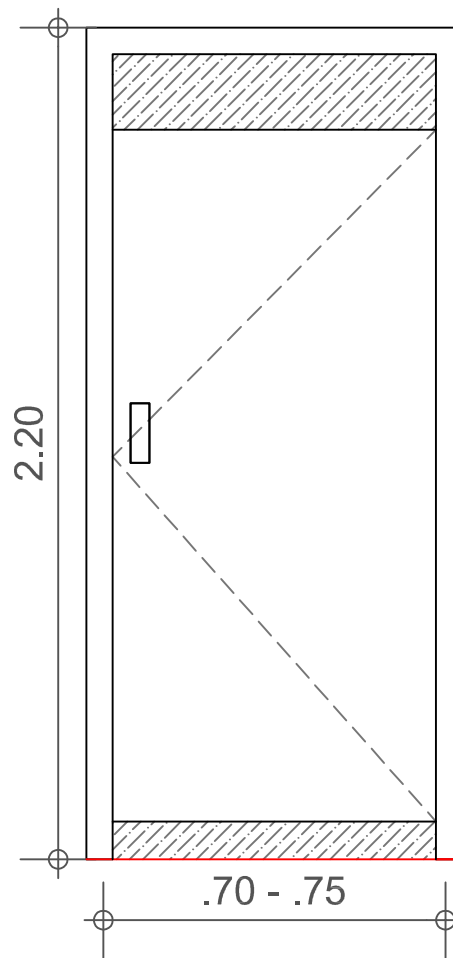
ΘΥΡΑ WC / ΑΚΑΘΑΡΤΩΝ - ΤΕΜ.3
