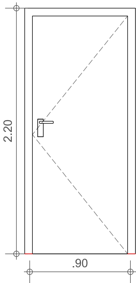
ΠΥΡΑΝΤΟΧΗ ΘΥΡΑ - ΤΕΜ.1
