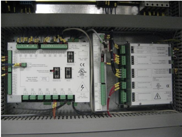
Φωτογρ.5: Ελεγκτής (controller) H/Z 1 (εντός ηλ. πίνακα)
