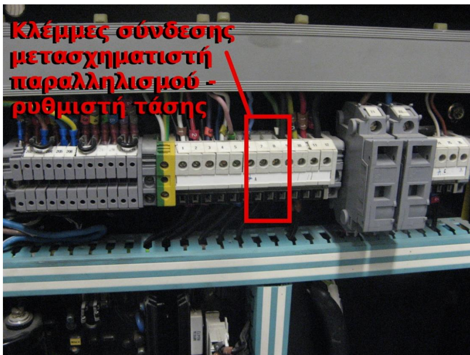
Φωτογρ.11: Κλεμμοσειρά H/Z (εντός του ερμαρίου ηλεκτρικών του H/Z)
