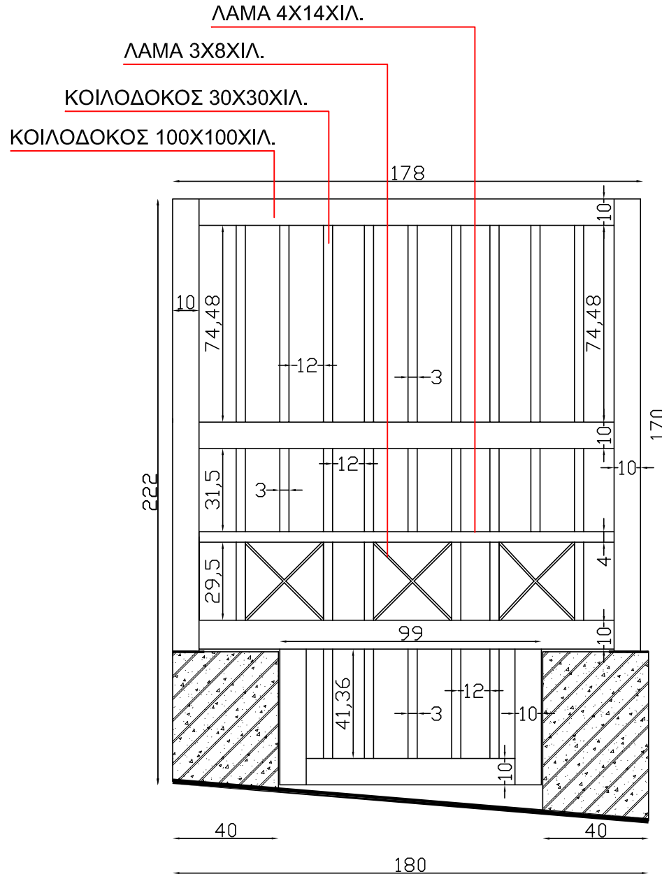
ΠΡΟΤΑΣΗ ΔΙΑΜΟΡΦΩΣΗΣ ΕΙΣΟΔΟΥ - ΟΨΗ - ΚΛ.1:20
