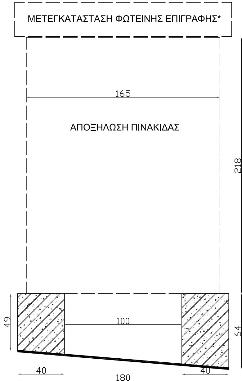
ΥΠΑΡΧΟΥΣΑ ΚΑΤΑΣΤΑΣΗ - ΟΨΗ - ΚΛ.1:20
